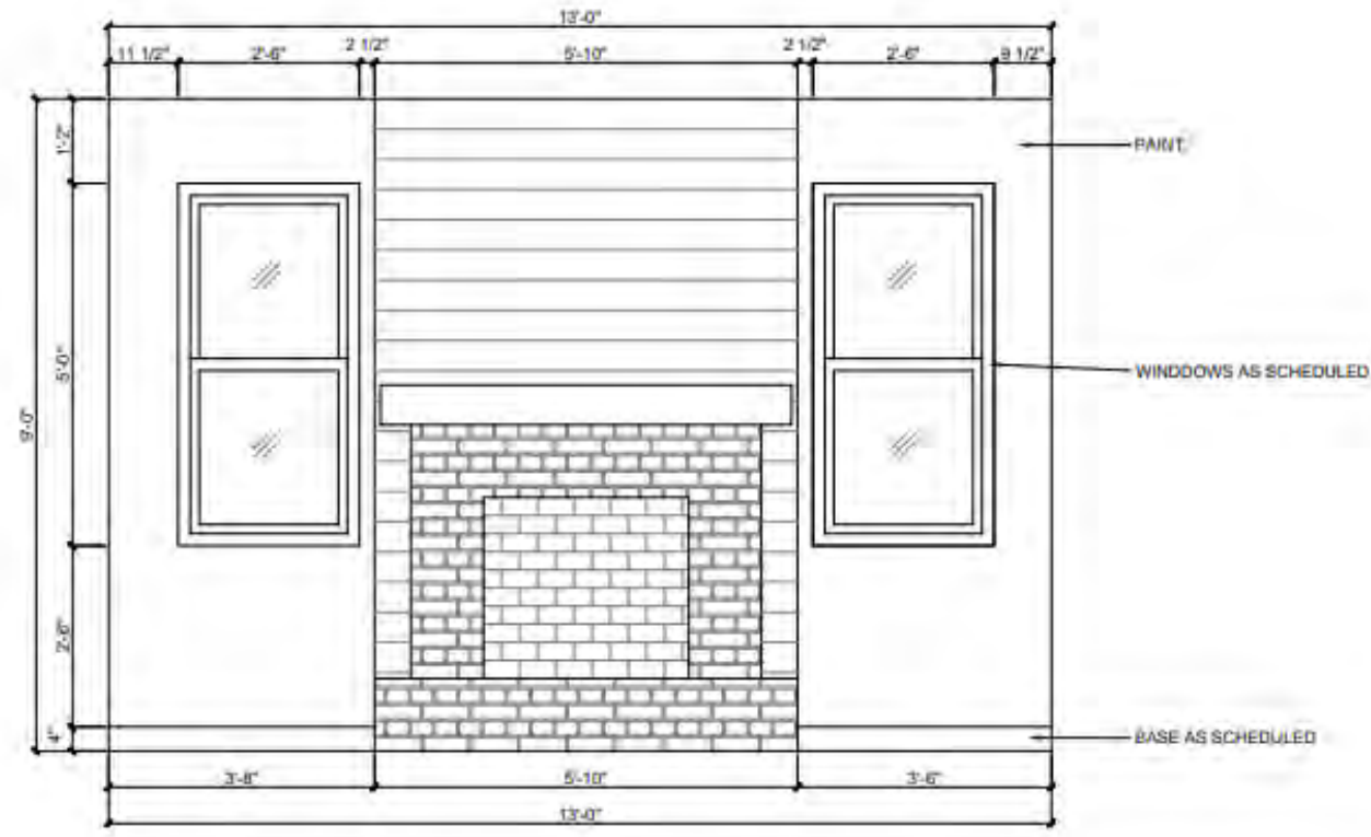
C FIREPLACE ELEVATION SCALE: 3/8" = 1'-0"
