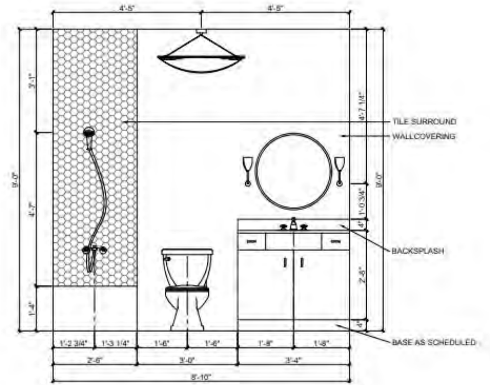
C BATHROOM ELEVATION SCALE: 3/8" = 1'-0"
