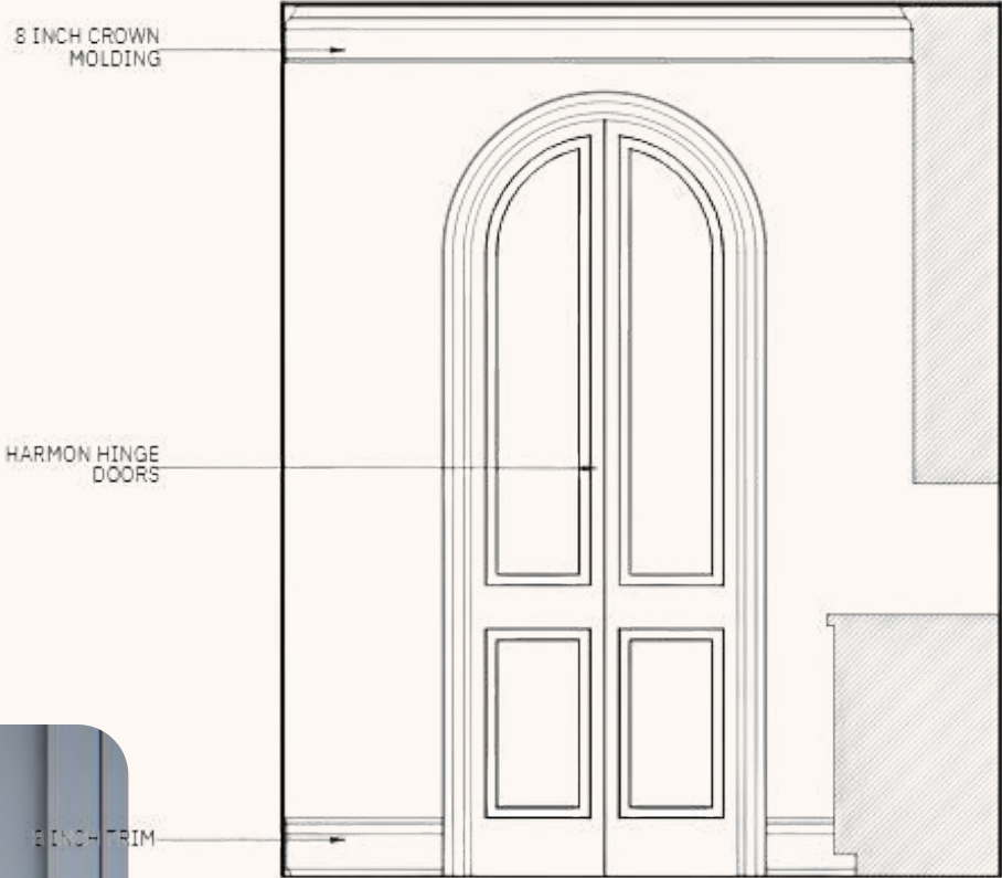
J. Sculler Door Elevation
