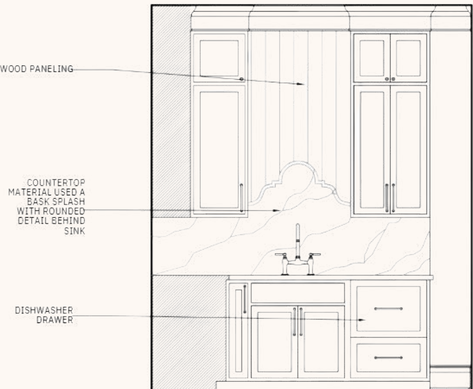
L. Scullery Sink Elevation
