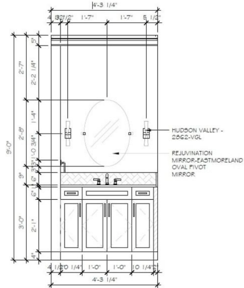
Elevation I
