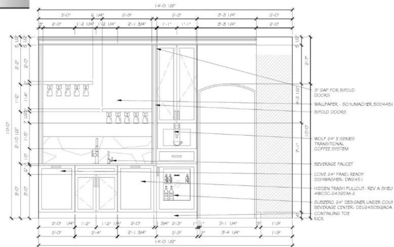
Elevation B
