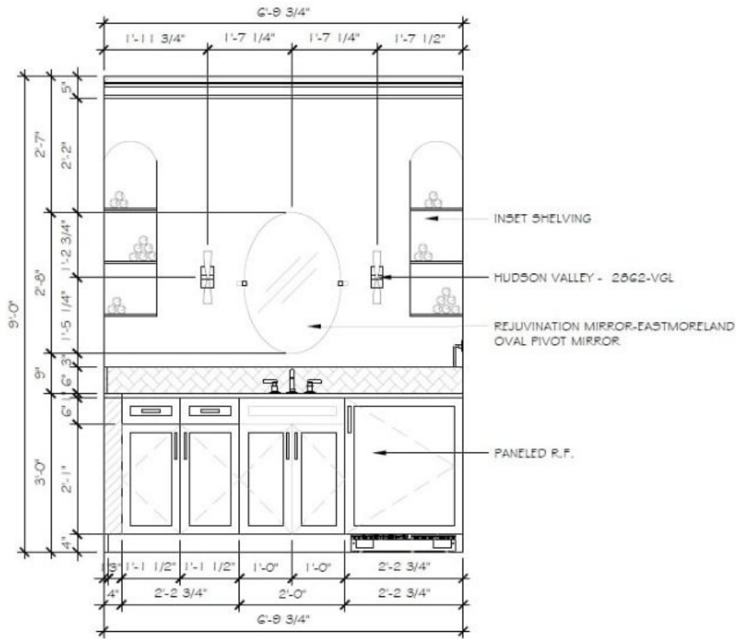
Elevation J
