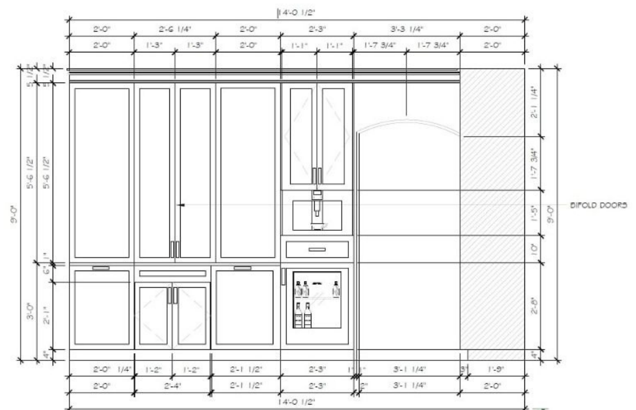
Elevation B
