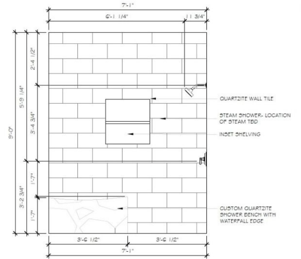
Elevation L
