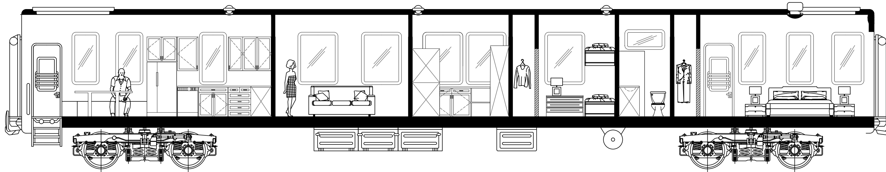
02 BACK SECTION SCALE: 3/16" = 1'-0"
