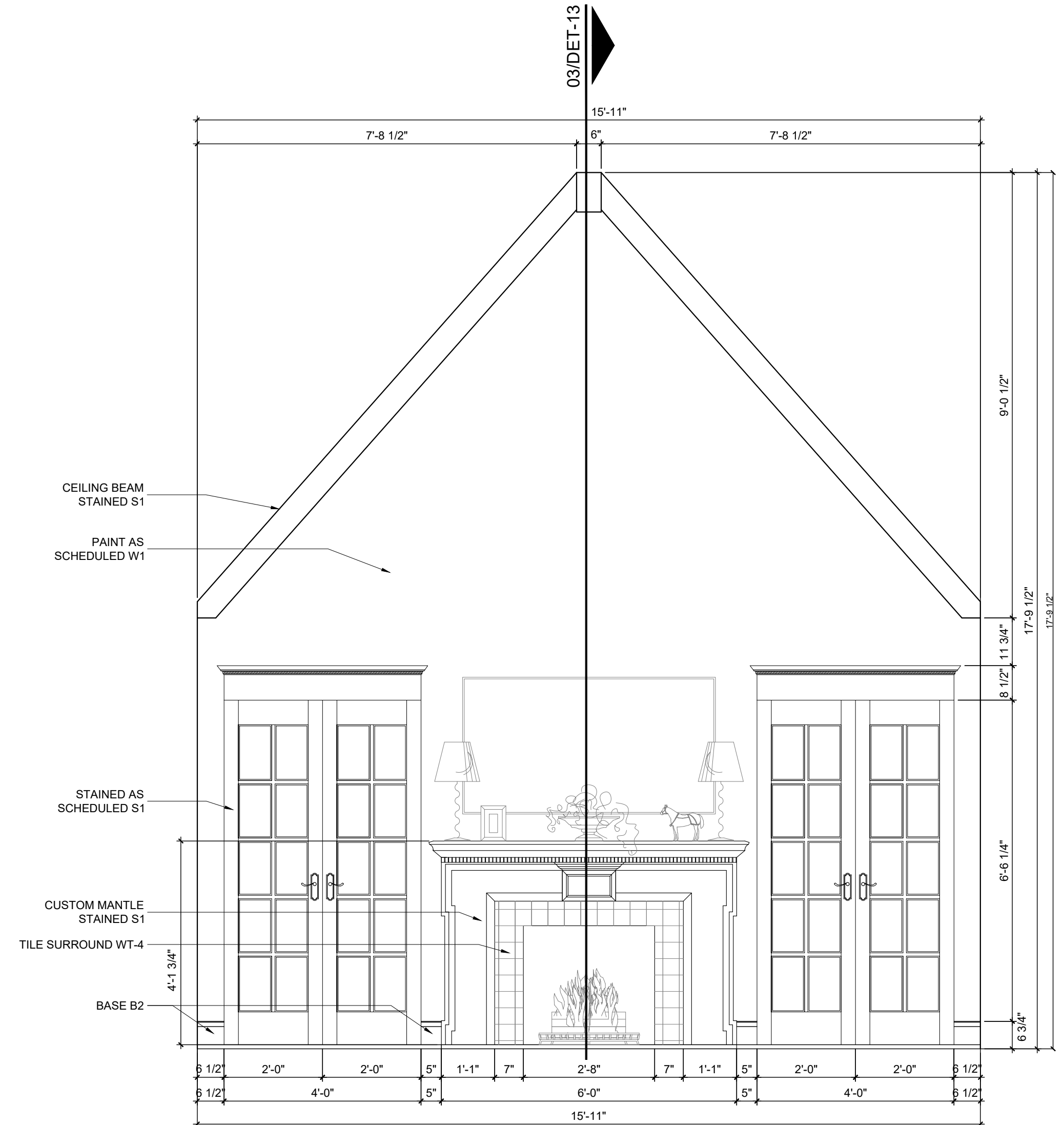
G FIREPLACE ELEV. SCALE: \frac{1}{2}" = 1' - 0"
