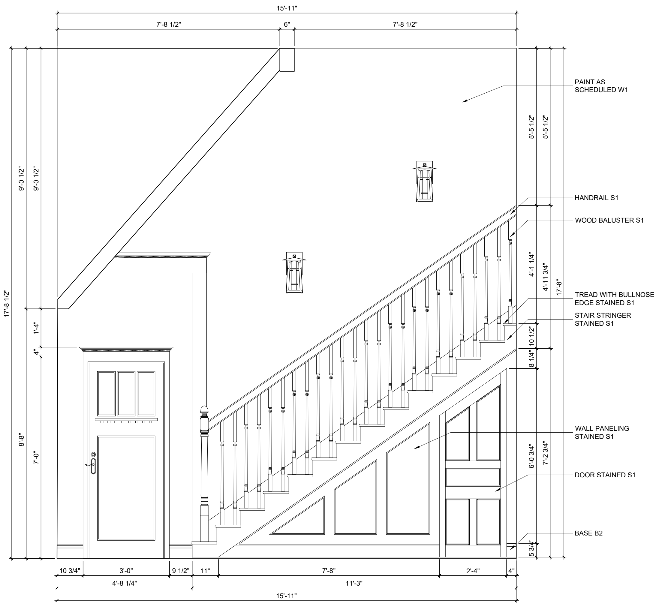
F STAIR ELEVATION SCALE: \frac{1}{2}" = 1'-0"
