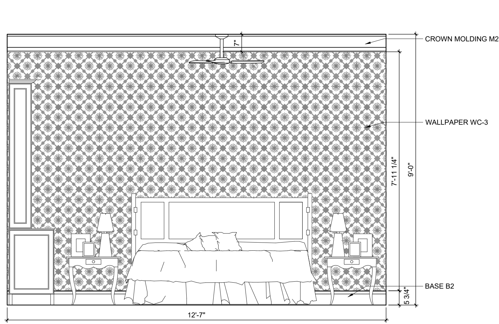
L MASTER BEDROOM ELEV. SCALE: \frac{1}{4}" = 1' - 0"
