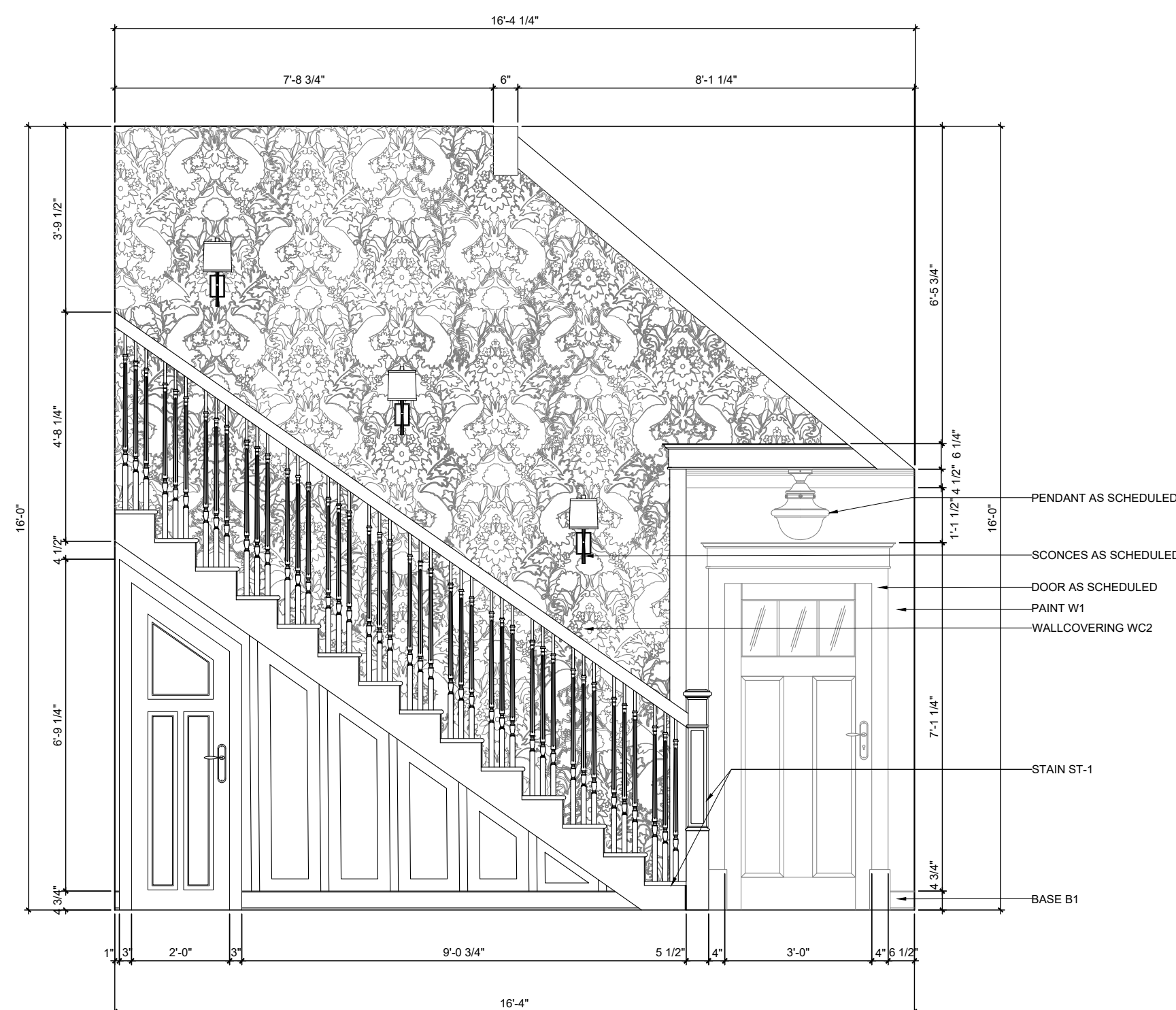
G STAIR ELEVATION SCALE: \frac{1}{8}" = 1' - 0"
