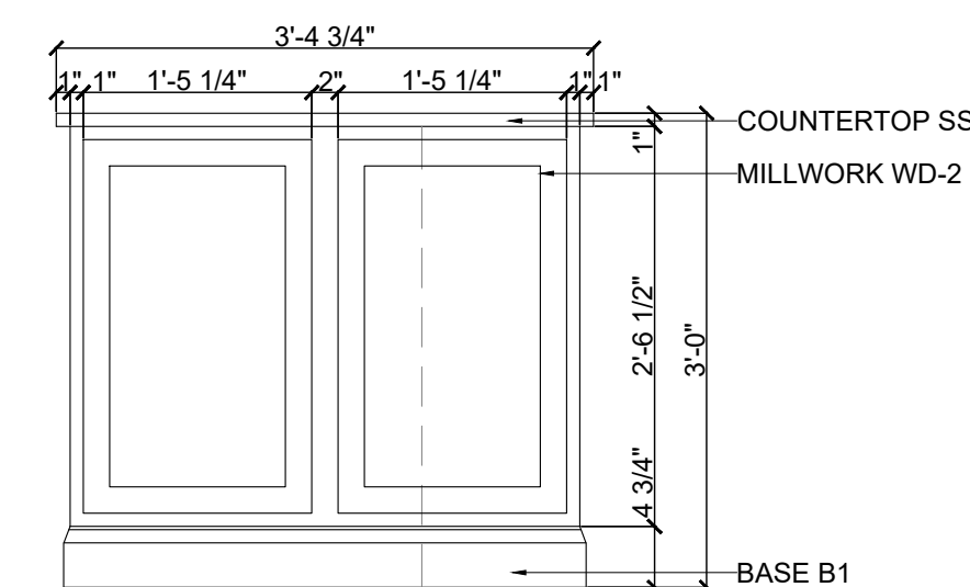
E SIDE ISLAND ELEV. SCALE: \frac{1}{8}" = 1' - 0"
